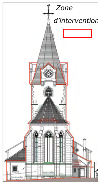
Élévation Est (doc. remis) Fabien Michel, Architecte du patrimoine - Maître d'Oeuvre
